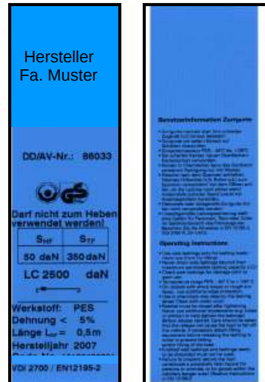
Abb. 20: Etikett nach EN 12195-2
